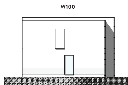
RECHTERGEVEL
