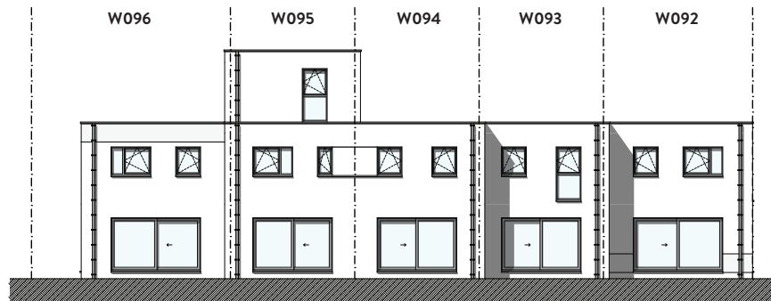
ACHTERGEVEL
