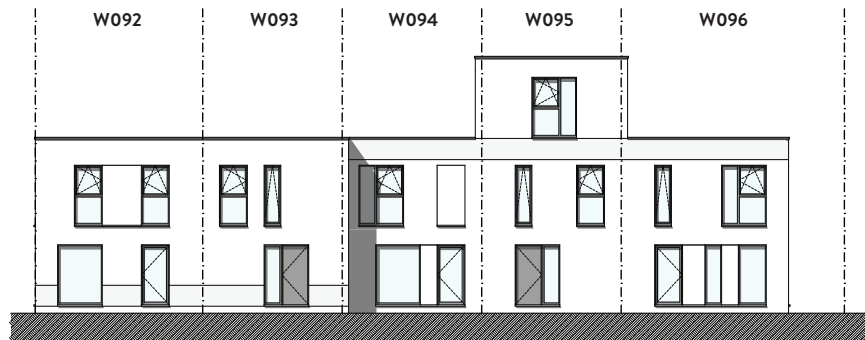
VOORGEVEL
