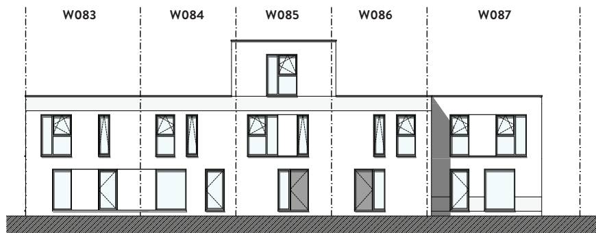
VOORGEVEL
