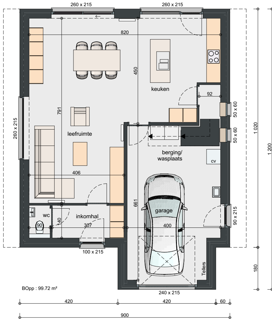
Gelijkvloers 1:100
