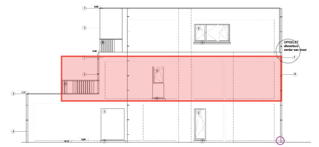
ZIJGEVEL LINKS
