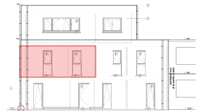
VOORGEVEL
